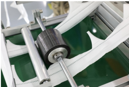
料片剥离装置 Piece peeling off device
